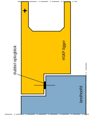
Oplegdetail landhoofd (tandoplegging)
