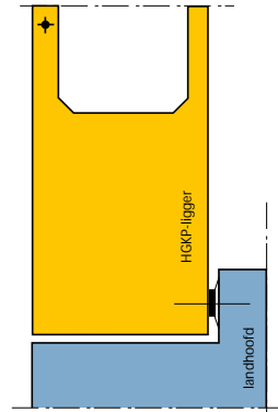
Oplegdetail landhoofd
