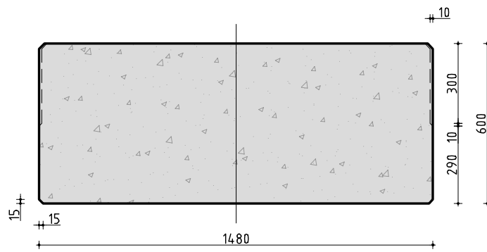
Doorsnede HKP600-ligger
