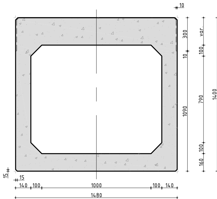
Doorsnede HKP1400-ligger
