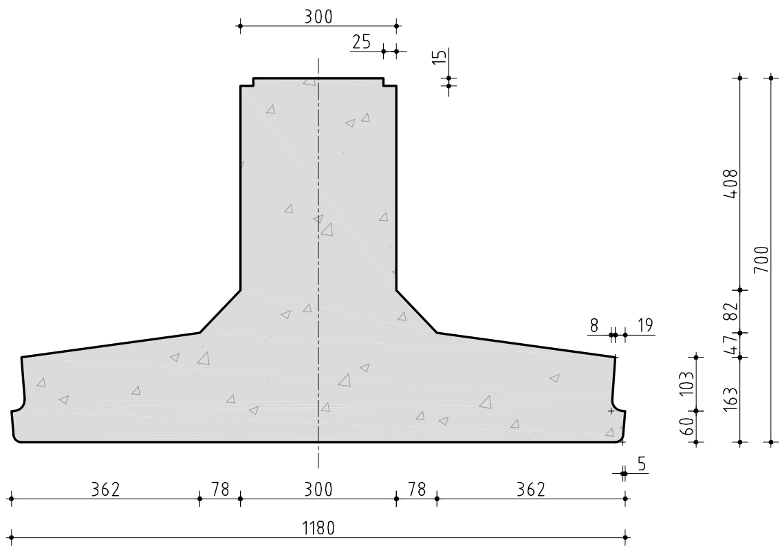
Doorsnede HRP-700-ligger
